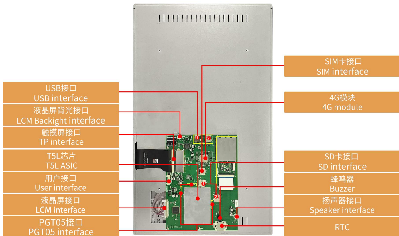
硬件接口图
