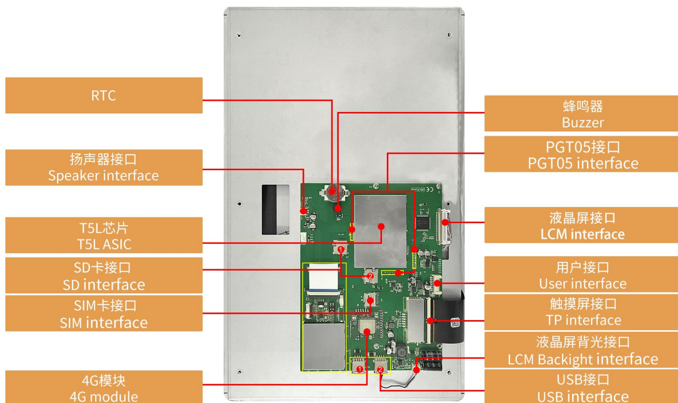
硬件接口图
