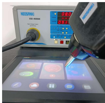
3.1 静电放电测试图 Electrostatic discharge test
