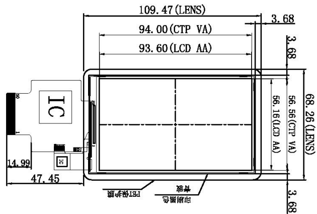
正视图
