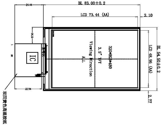
正视图
