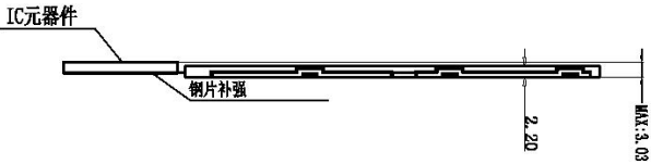
侧视图
