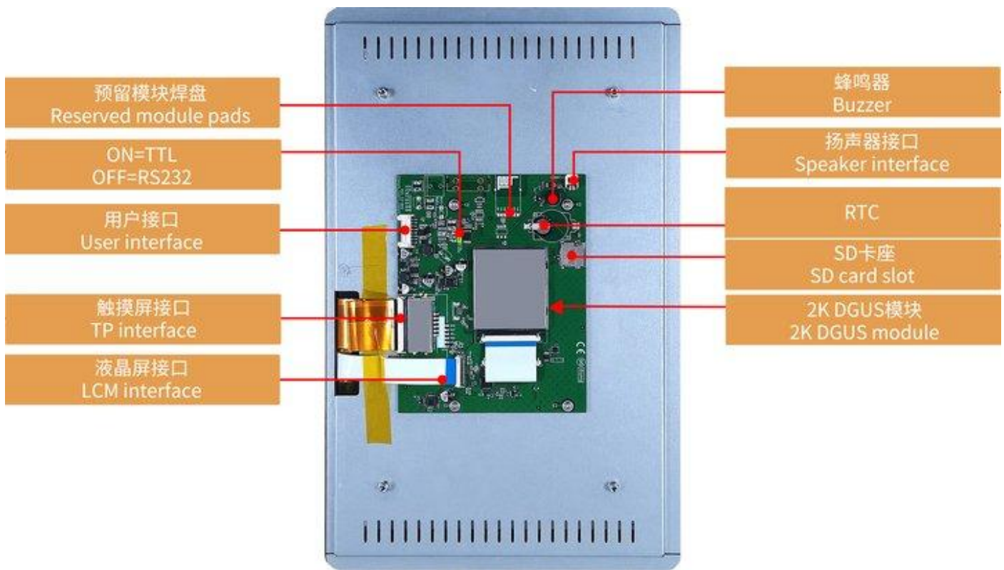
硬件接口图
